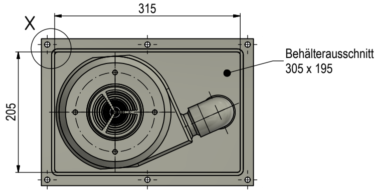
Ansicht A
